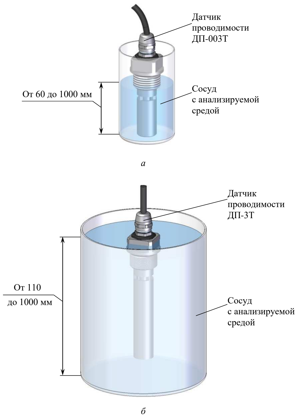
Рисунок 2.9 – Пример расположения датчика проводимости в сосуде с анализируемой средой при погружном способе измерений
