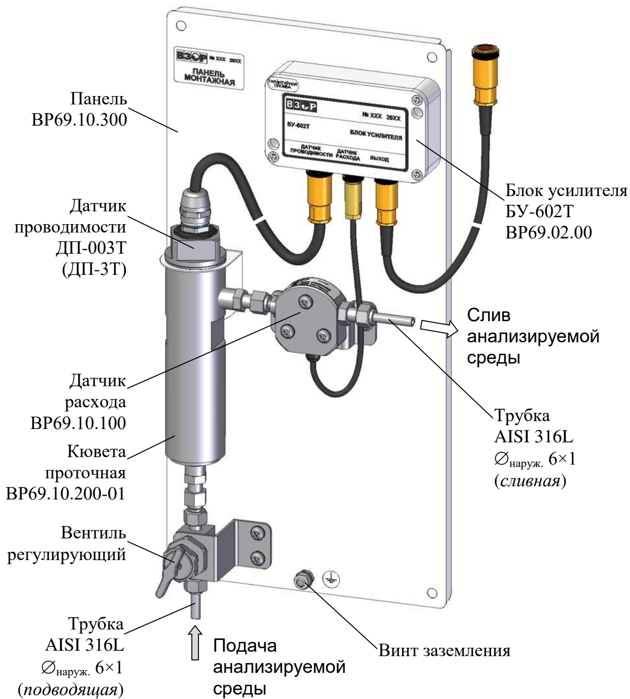
Рисунок 2.10 – Расположение датчика проводимости ДП-003Т (ДП-3Т) на панели монтажной ВР69.10.000 (проточный способ измерений)
