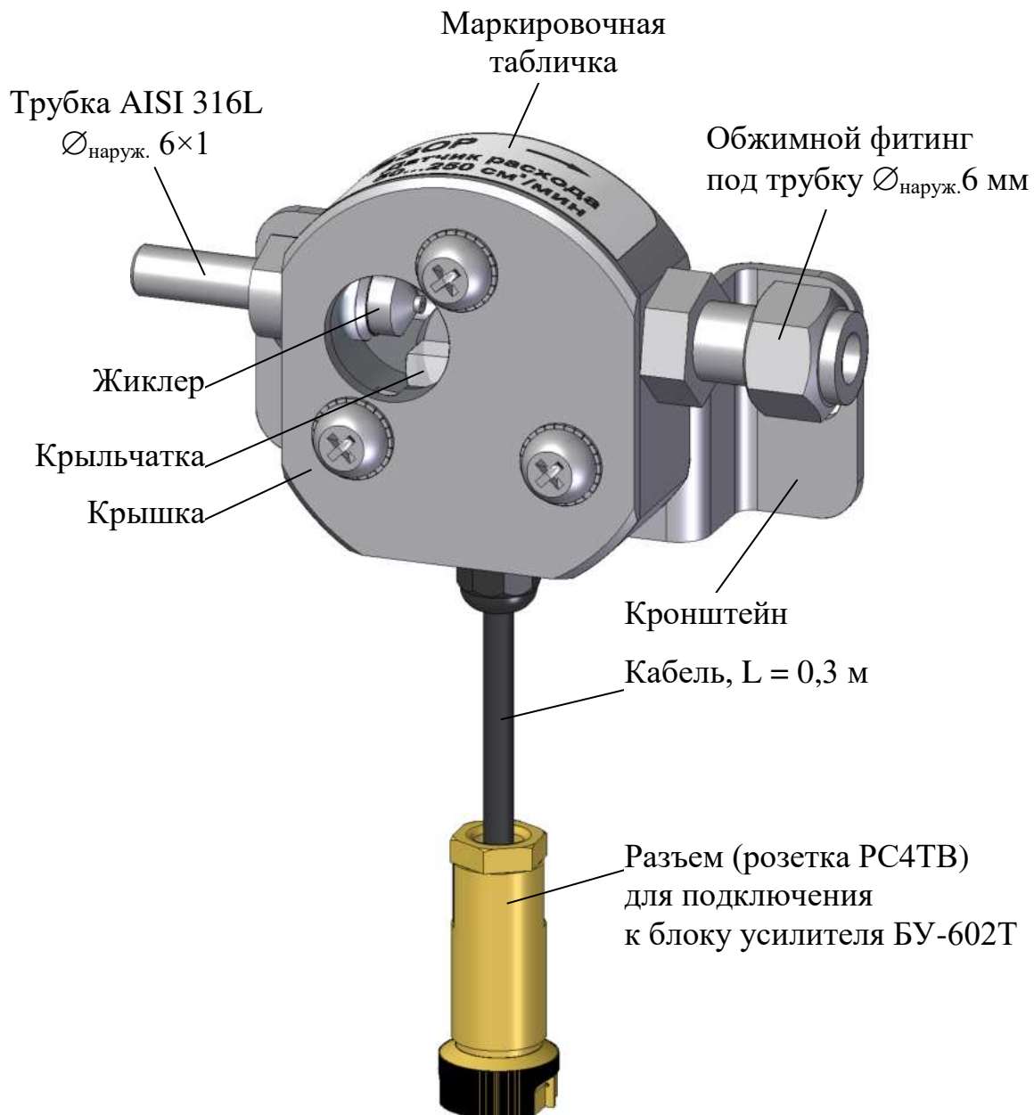
Рисунок 1.8 – Датчик расхода (вид с разрезом)
