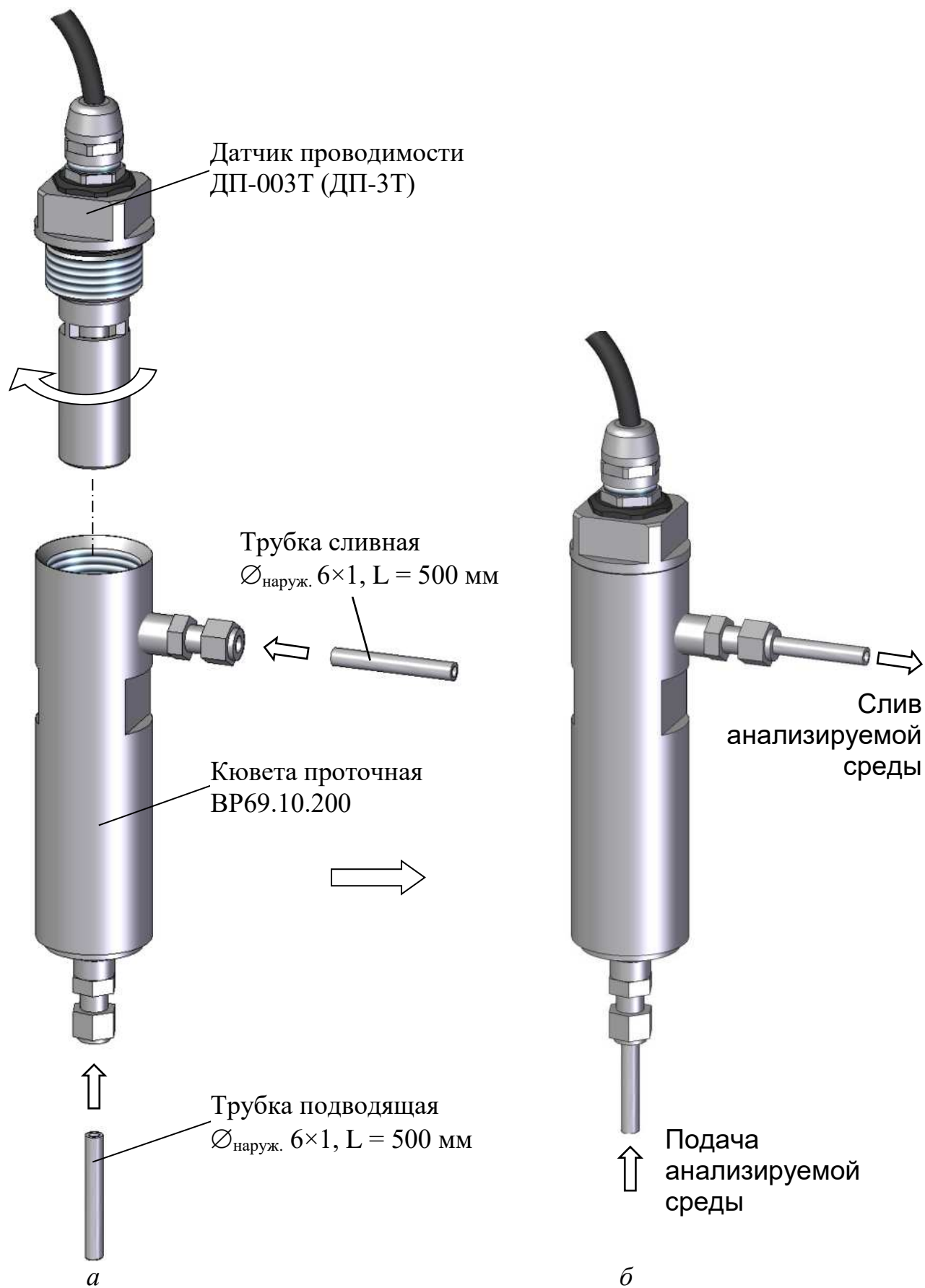
Рисунок 2.11 – Расположение датчика проводимости ДП-003Т в кювете проточной BP69.10.200 при проточном способе измерений
