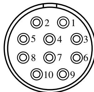
Розетка РС10ТВ (вид со стороны пайки контактов)
