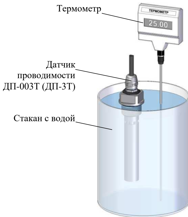
Рисунок 3.12 – Проверка показаний по температуре
