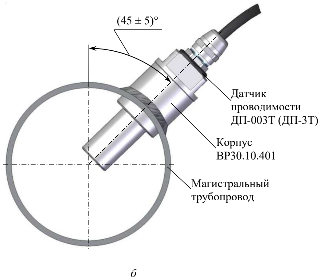
Рисунок 2.13 – Расположение датчика проводимости ДП-003Т (ДП-3Т) в магистральном трубопроводе
