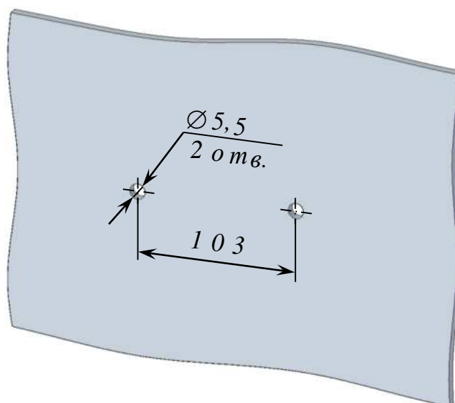
Рисунок 2.14 – Расположение и размер отверстий для крепления датчика расхода на панели монтажной ВР69.10.000
