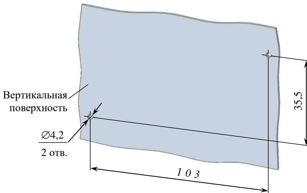
Рисунок 2.7 – Расположение и размер отверстий для крепления блока усилителя БУ-602Т
