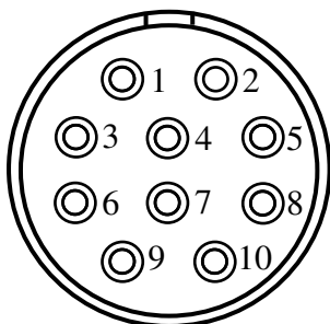
Вилка РСГ10ТВ (вид со стороны пайки контактов)
