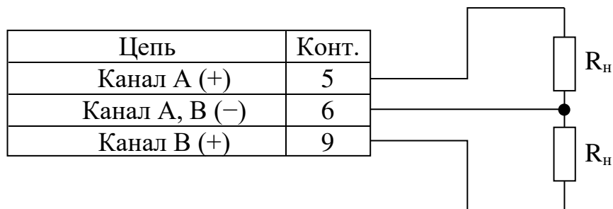
Рисунок 2.5 – Схема подключения внешней нагрузки к контактам разъема « ТОКОВЫЙ ВЫХОД »
