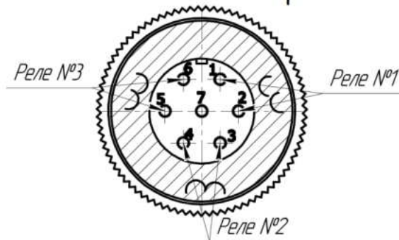
Рисунок 18 – Назначение контактов разъема MS-XS12-7PW/YS
