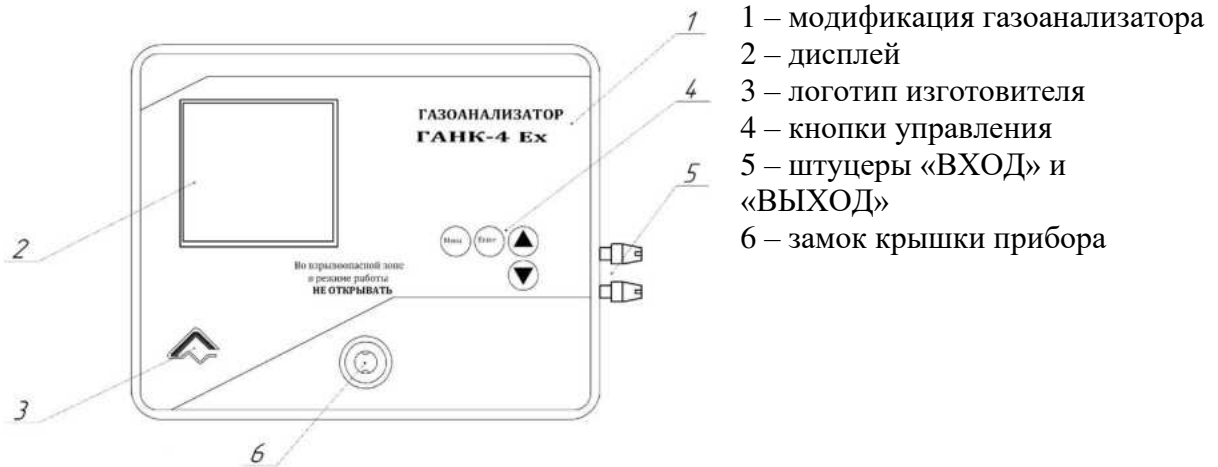
Рисунок 11 – Вид спереди
