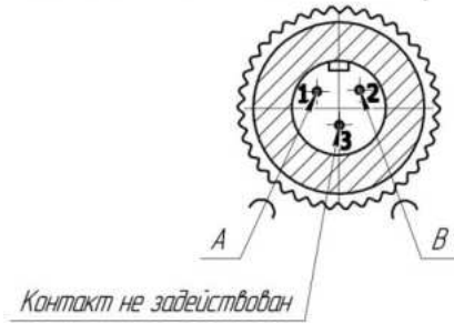
Рисунок 17 – Назначение контактов разъема MS-XS8-3PW/YS
