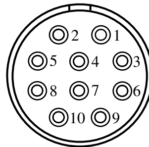
Розетка РС10ТВ (вид со стороны пайки контактов)
