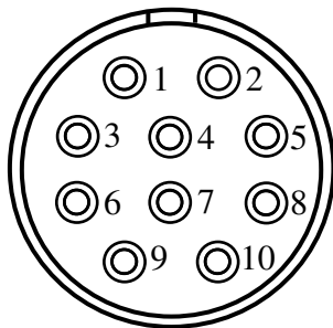
Вилка РСГ10ТВ (вид со стороны пайки контактов)
