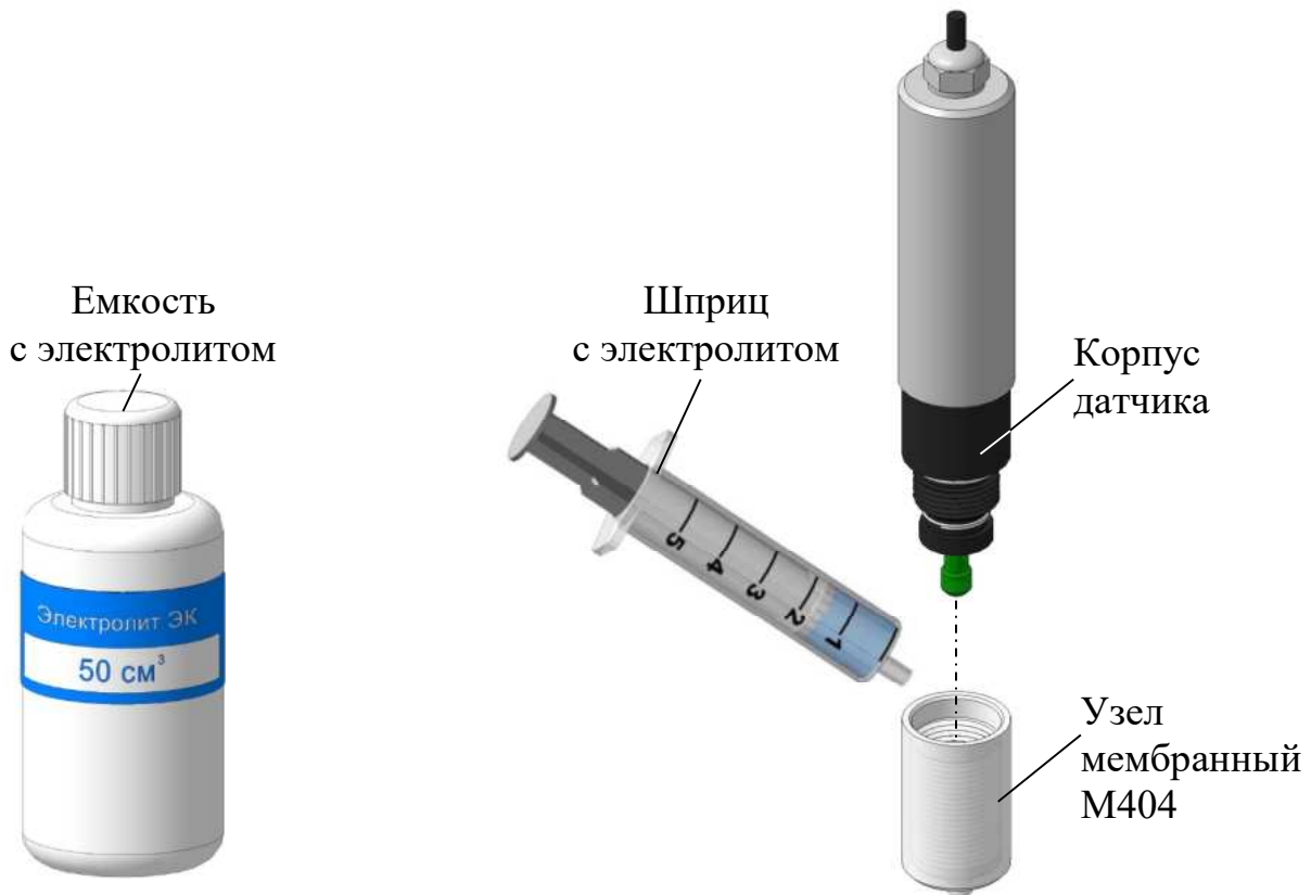
Рисунок 2.3 – Заливка (добавление) электролита ЭК
