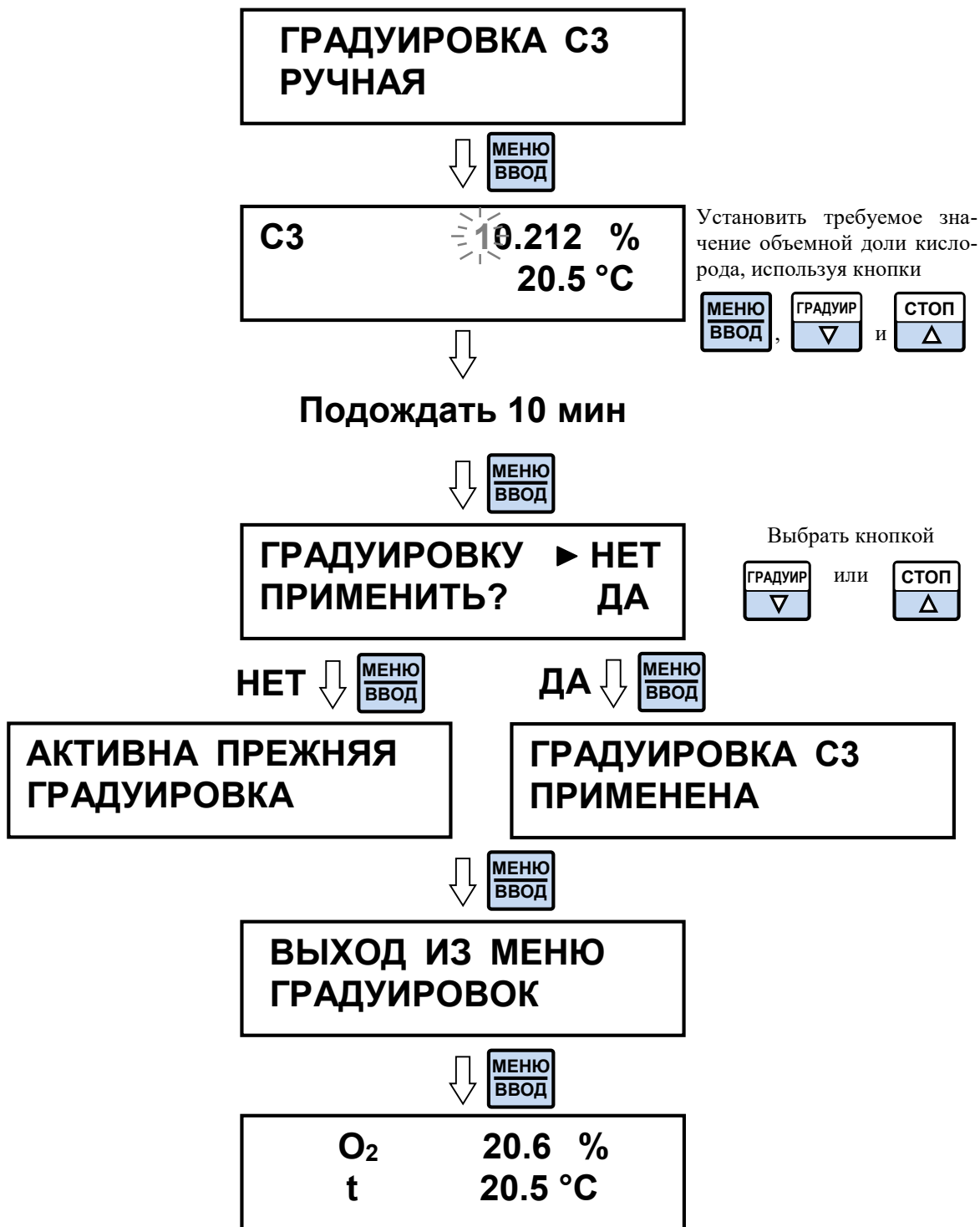
Рисунок 2.10 – Градуировка по ГСО-ПГС
