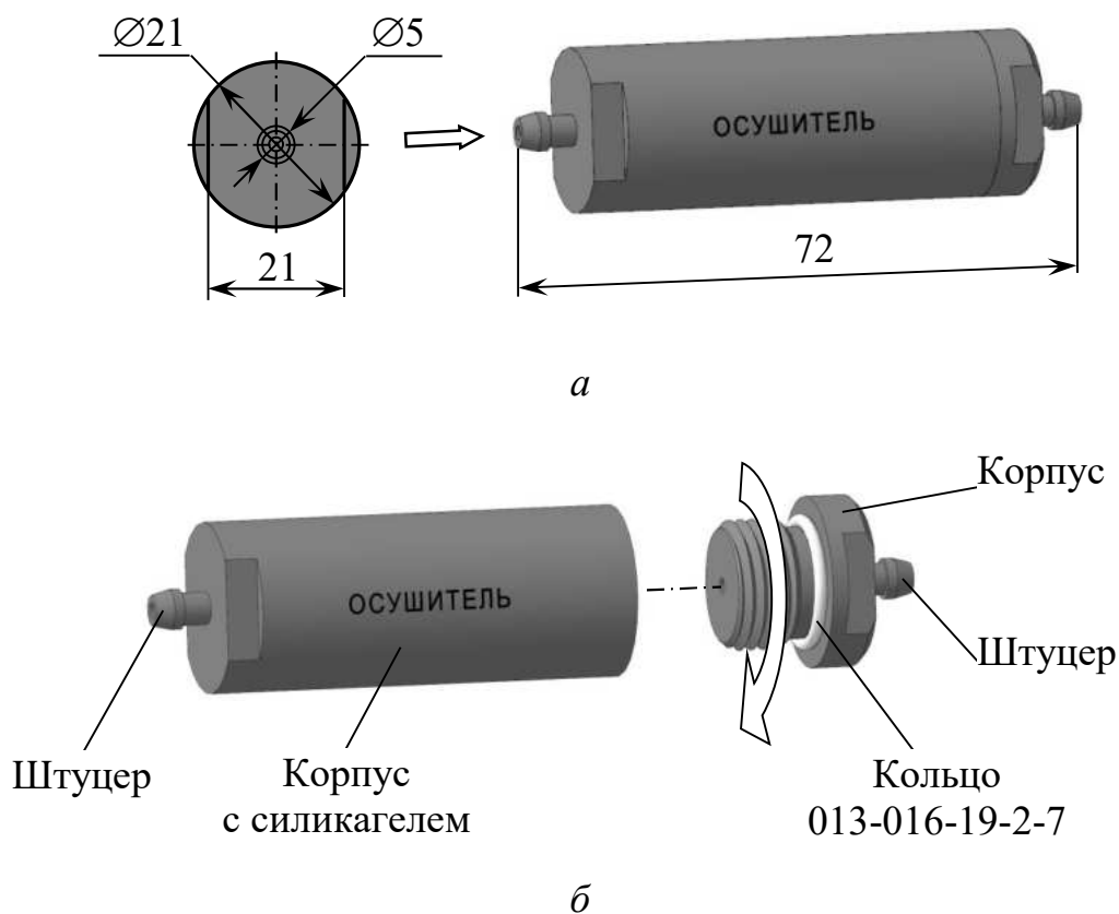
Рисунок 1.4 – Осушитель ВР84.04.120
