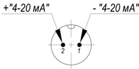
Рисунок 43 – Назначение контактов разъема MS-XS8JK-2PW/YS
