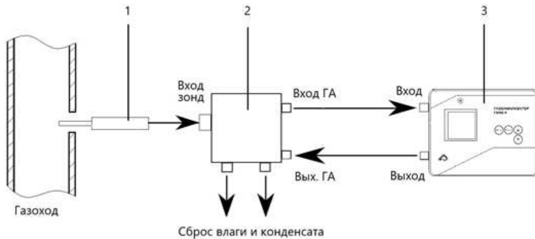
Рисунок 1 – Схема пробоотбора
