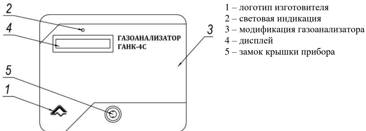
Рисунок 14 – Вид спереди
