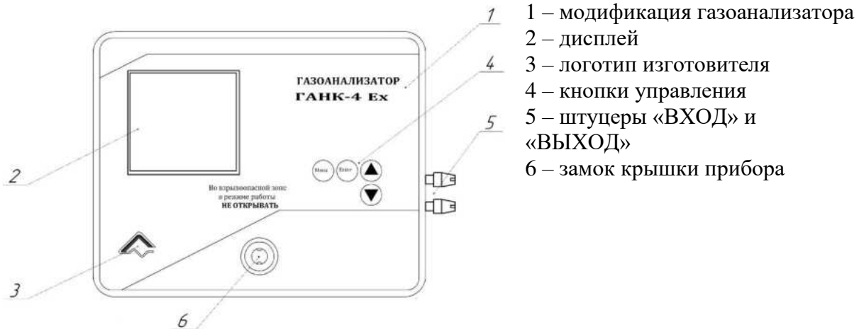
Рисунок 11 – Вид спереди
