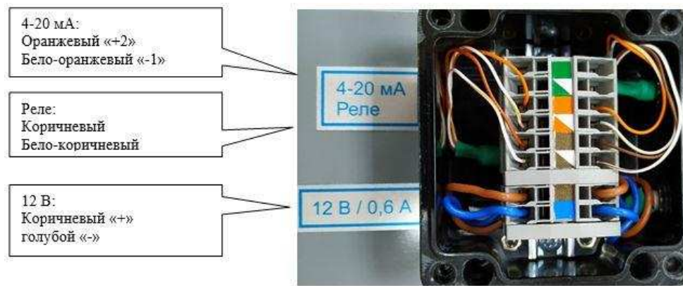
Рисунок 30 – Общий вид монтажной коробки газоанализатора ГАНК-4С Ex 12.9 Проведение измерений с использованием датчиков
