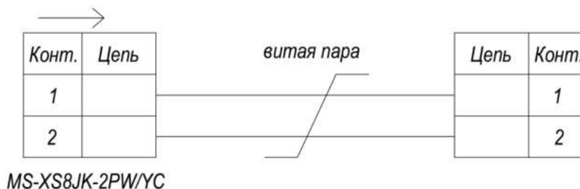
Рисунок 44 – Схема электрическая соединений разъема MS-XS8JK-2PW/YS
